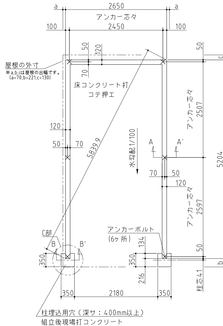
基礎詳細図 S=1/20
